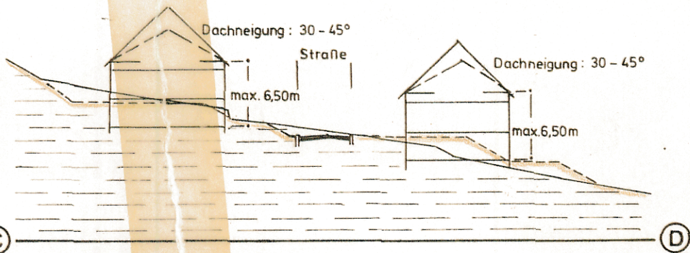
Regelschnitt Maßstab 1: 500
