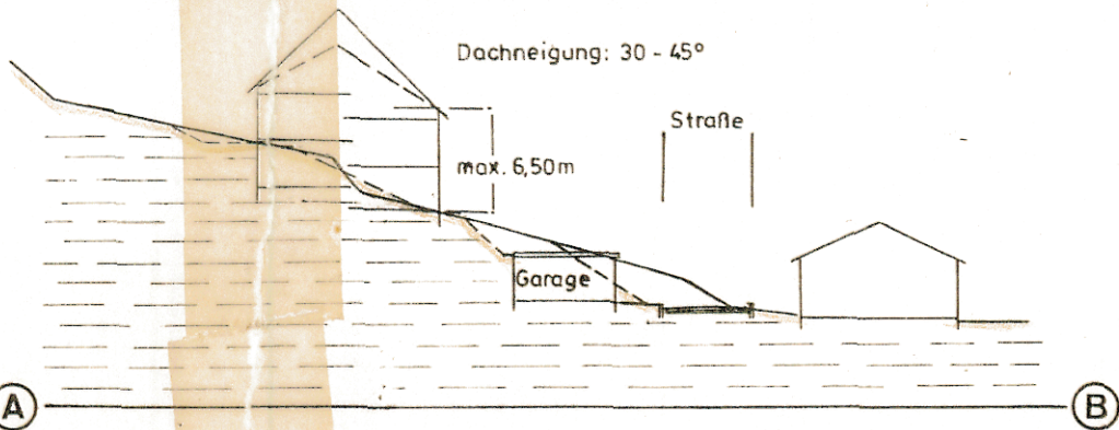
Regelschnitt Maßstab 1: 500
